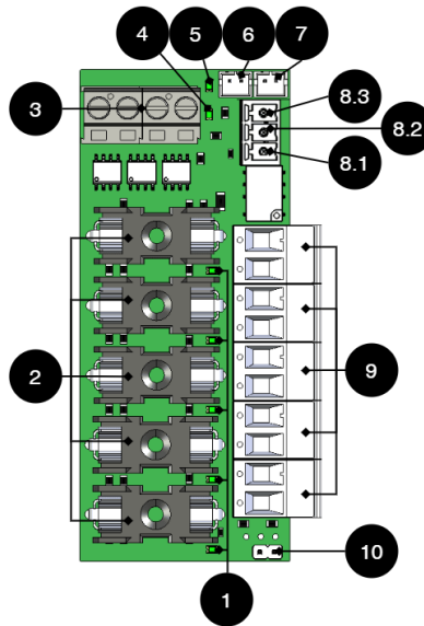
Taulu 16. Piirilevyn yleiskatsaus - BT FUSE 5
