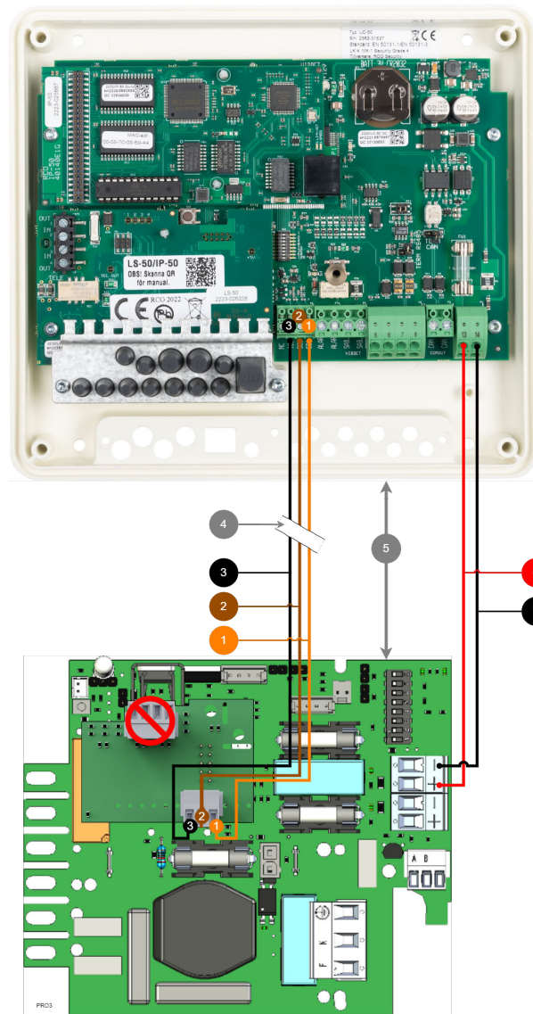
Kuva 4. Liitäntä UC-50 Gen2:een
