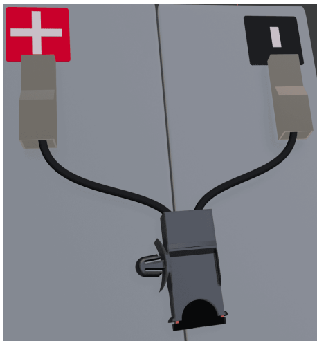
Figur 1. Sikringsholder med flatstiftsikring kobles til pluss og minus på batterier
