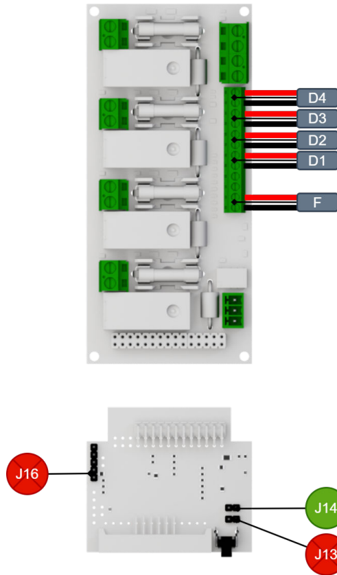
Taulu 7. Puserot negatiivisella logiikalla - yksilöllinen ohjaus.
