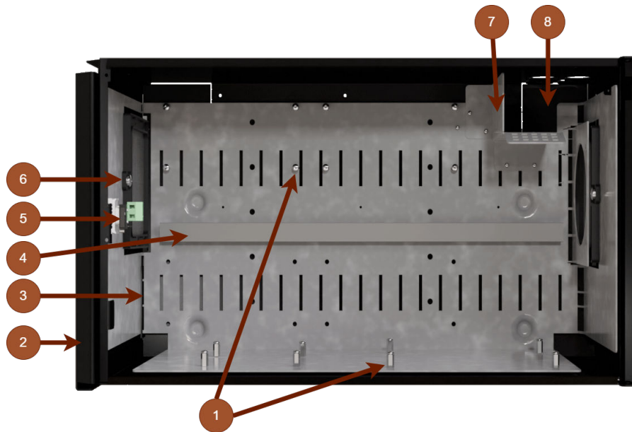
Bild på hur komponenter kan monteras.
